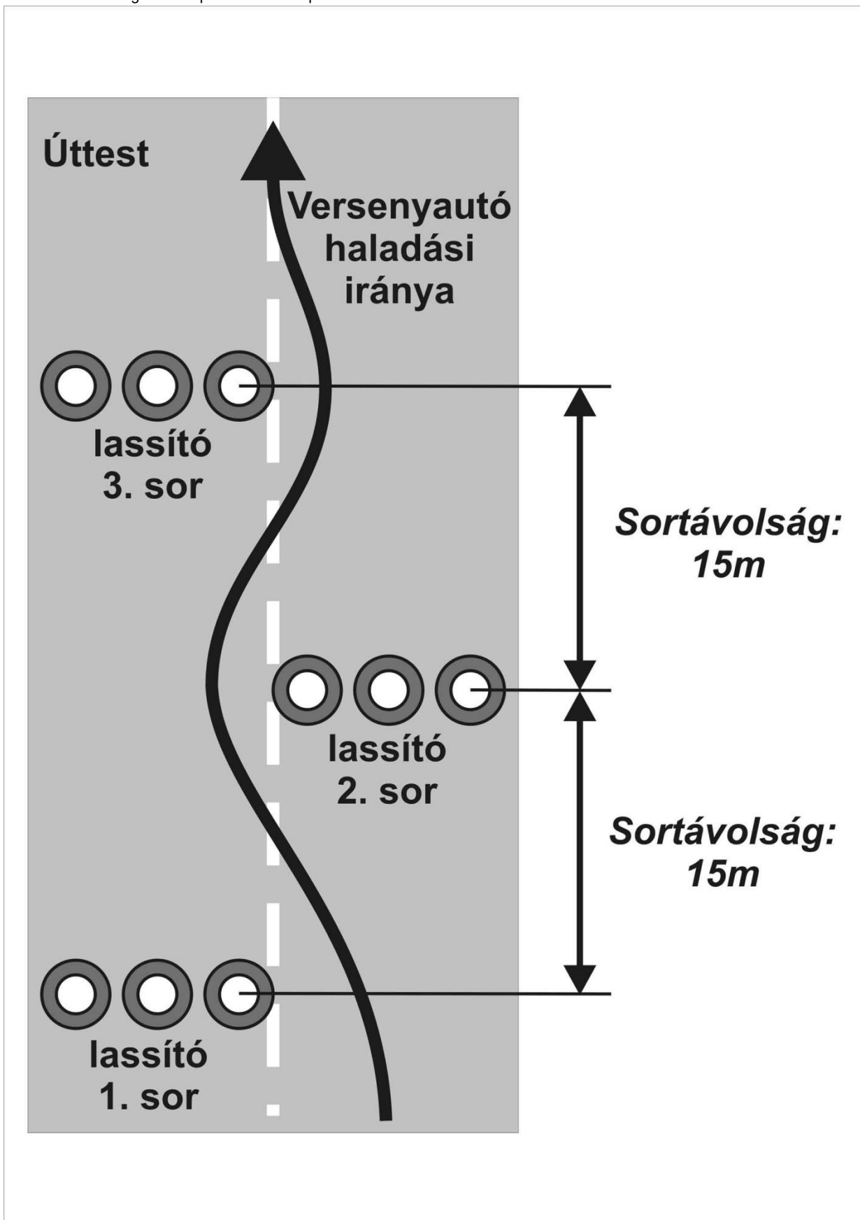
4. ábra: A mesterségesen telepített lassító felépítése
